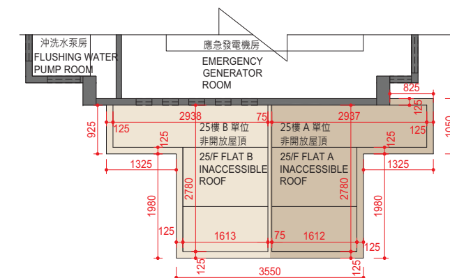
UPPER ROOF PART PLAN 上層天台局部平面圖
